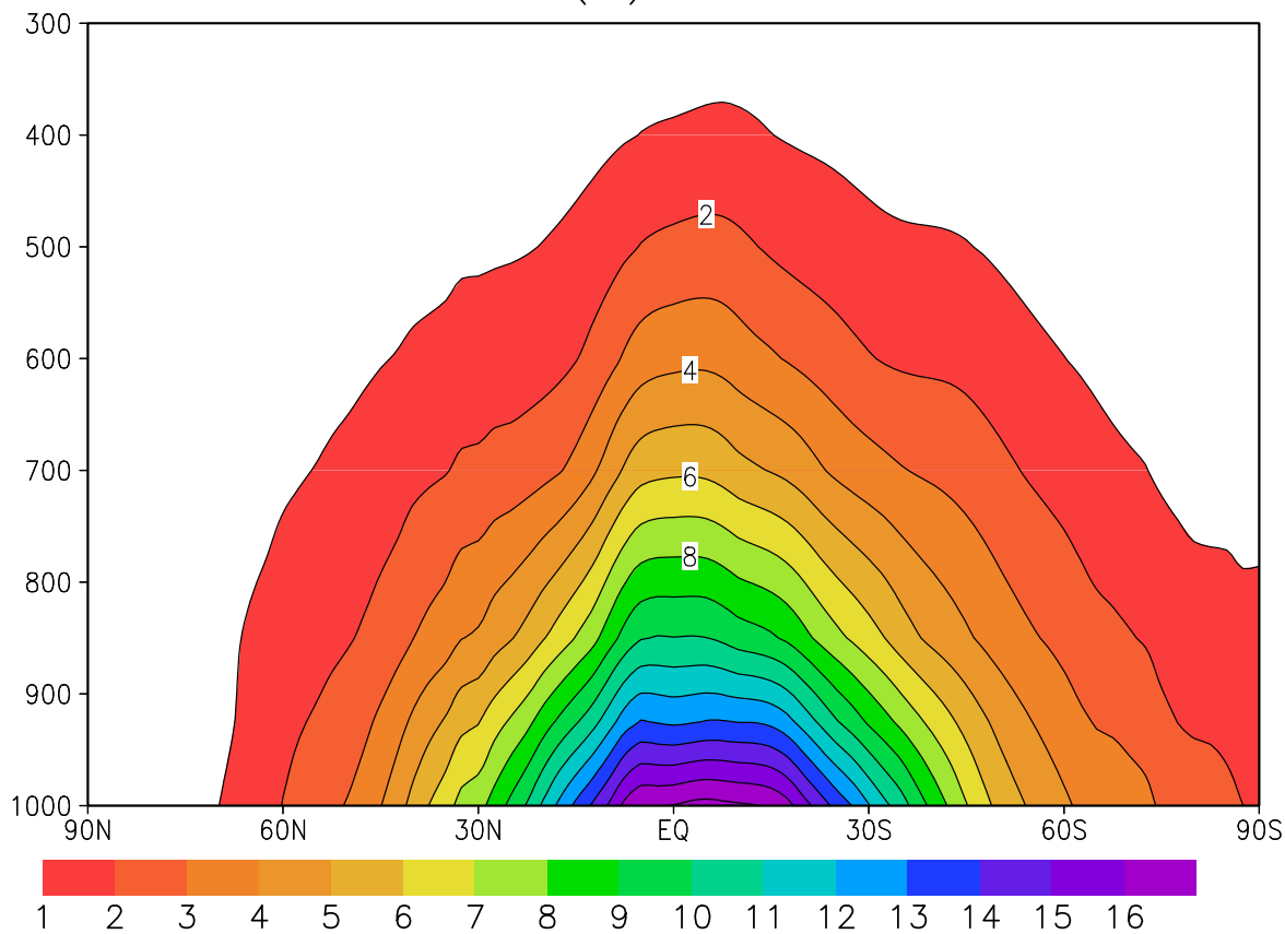
(a) DJF
